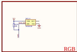
RGB
