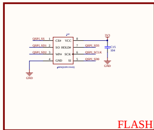
FLASH
