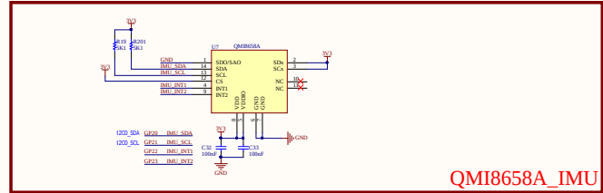
QMI8658A_IMU
