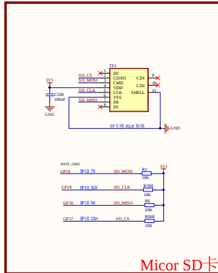
Micor SD卡
